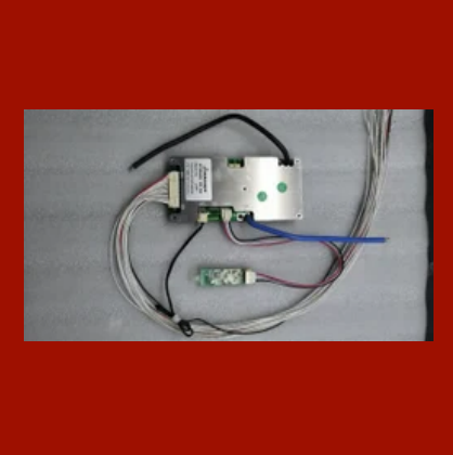
15S/40A Lifepo4 Smart BMS
